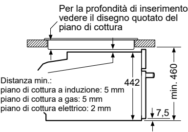
Montaggio con un piano di cottura.
