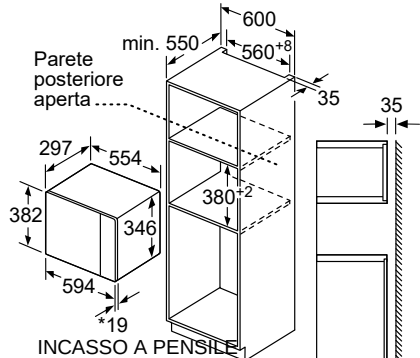
INCASSO A COLONNA
