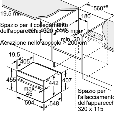
INCASSO SOTTOPIANO
