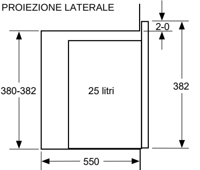
PROIEZIONE LATERALE
