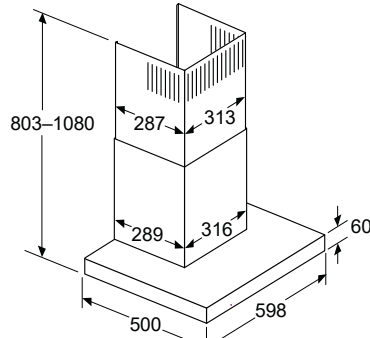
Prospettiva ricircolo
