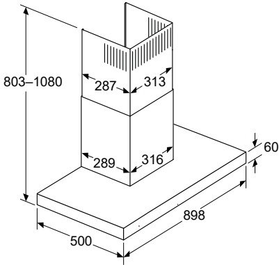
Prospettiva ricircolo
