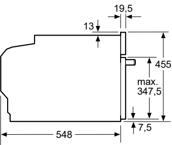
PROIEZIONE LATERALE
