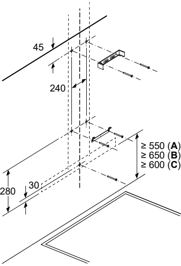
Installazione a parete con camino
