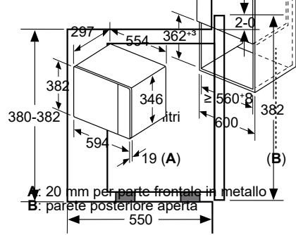
INCASSO A PENSILE
