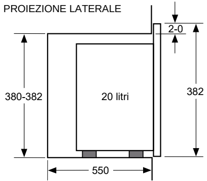
PROIEZIONE LATERALE
