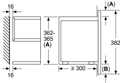
INCASSO A COLONNA
