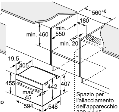
INCASSO SOTTOPIANO
