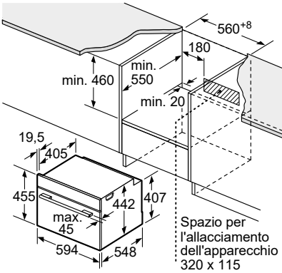
INCASSO SOTTOPIANO
