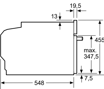
PROIEZIONE LATERALE
