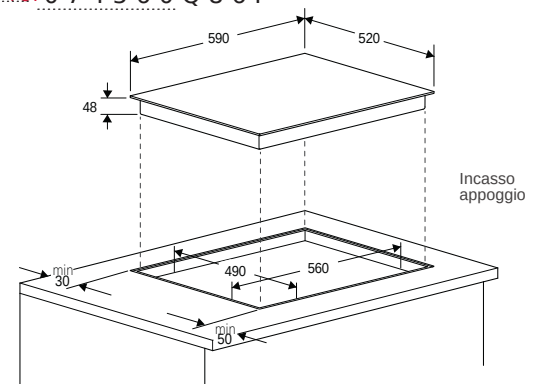
Schemi per incasso filo top da pagina 70
