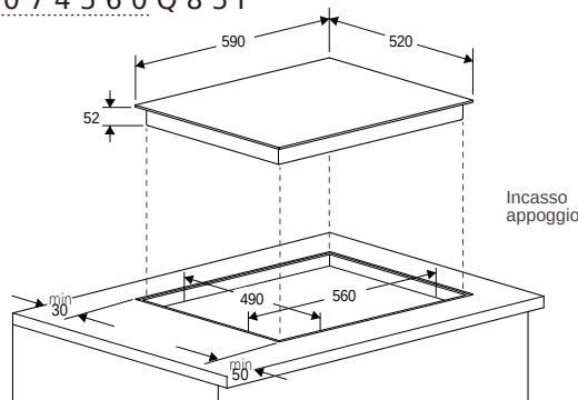
Schemi per incasso filo top da pagina 70
